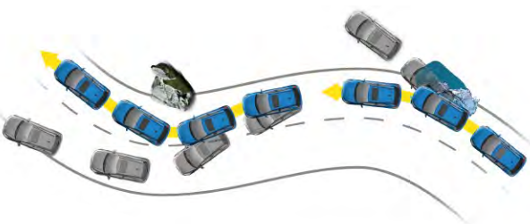
Układ ESC z układem VSM
